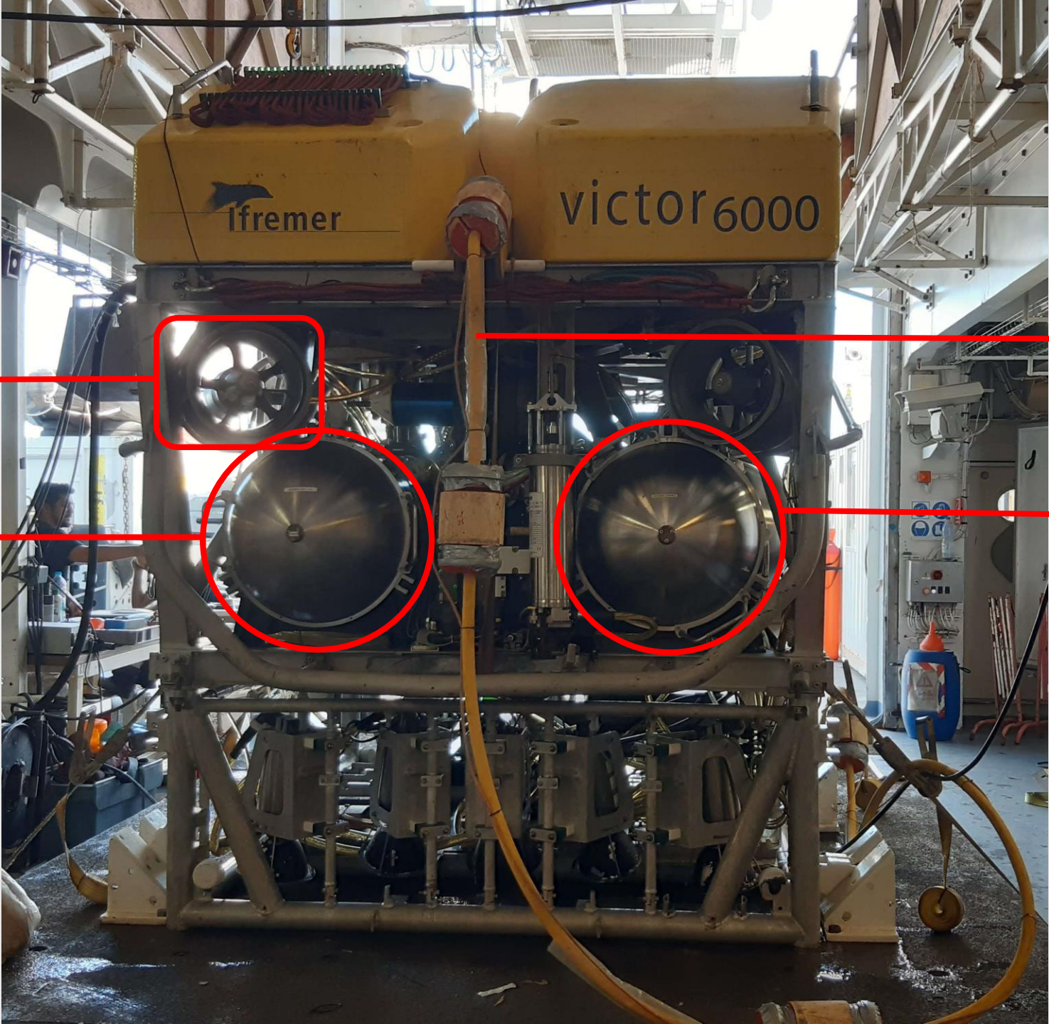
Face arrière du ROV Victor 6000
